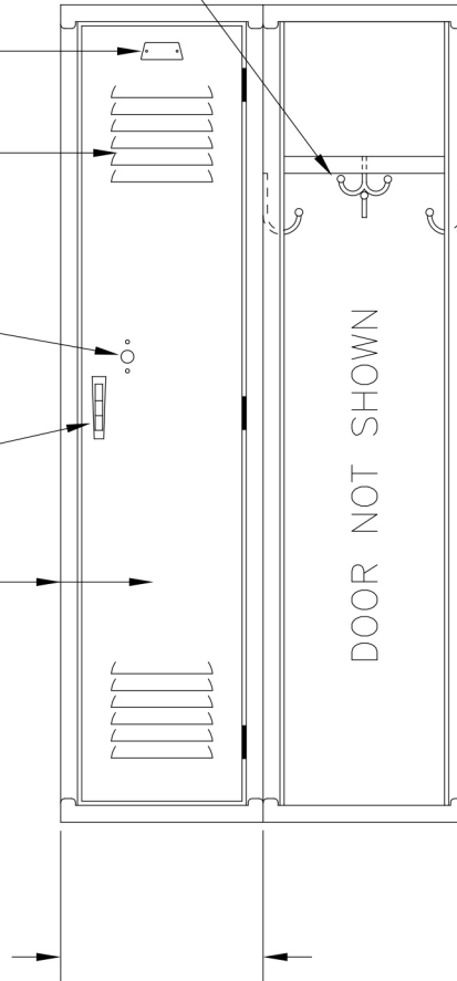
ELEVATION
