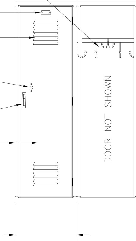
ELEVATION
