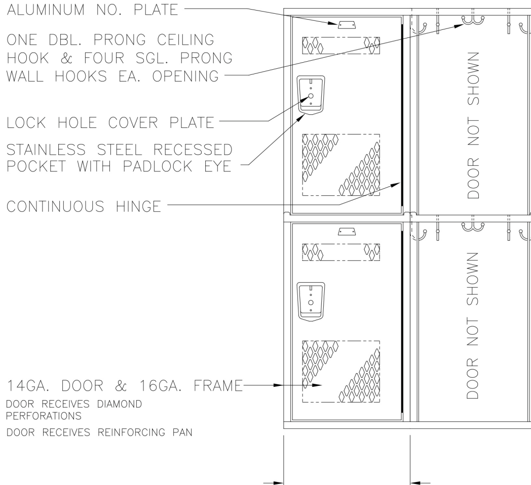
ELEVATION
