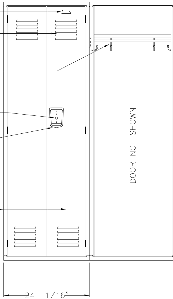
ELEVATION
